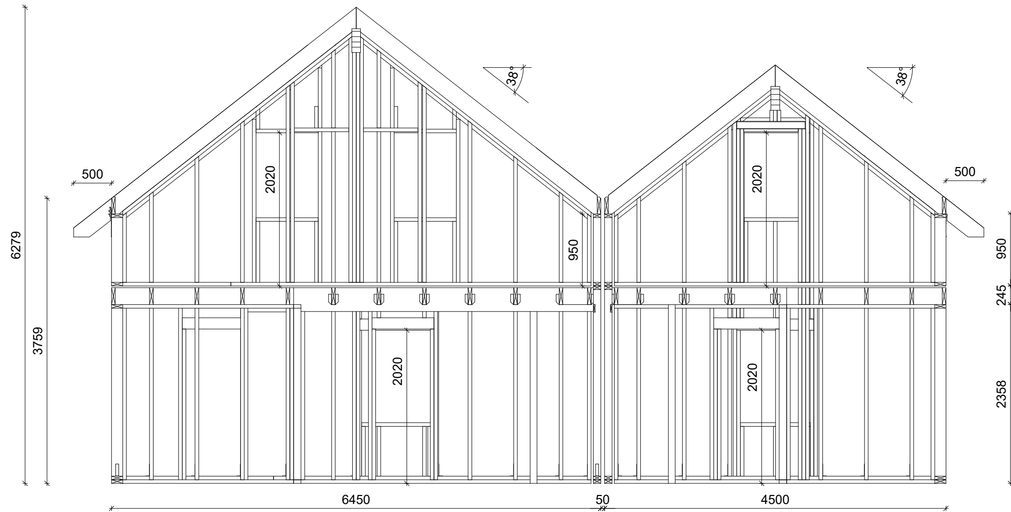
Snitt A-A
